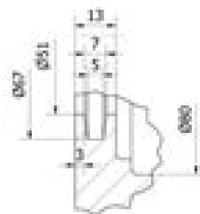
B (1 : 1)
