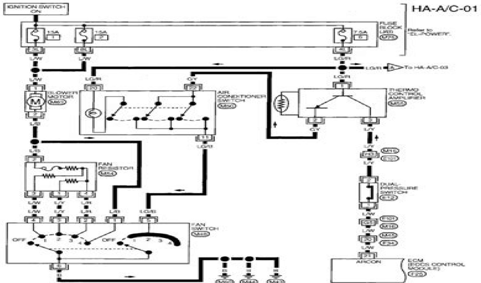
Wiring Diagram –A/C–
