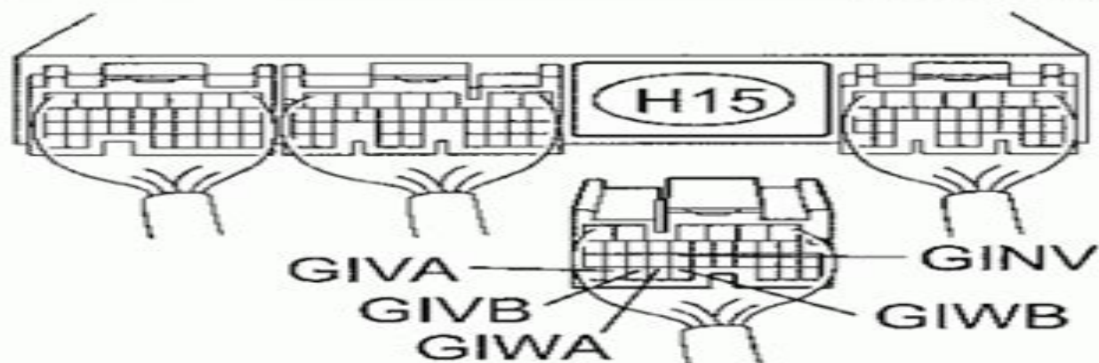
Y HV Control ECU Connector
