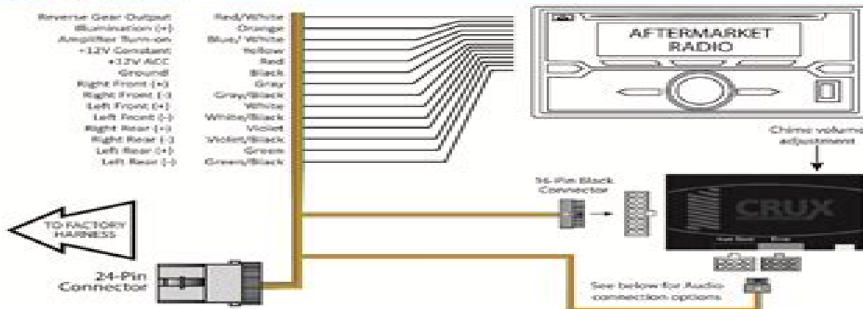
SDCGM-17C Module
