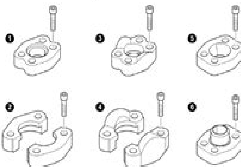
Fig. 1 SAE flanges
