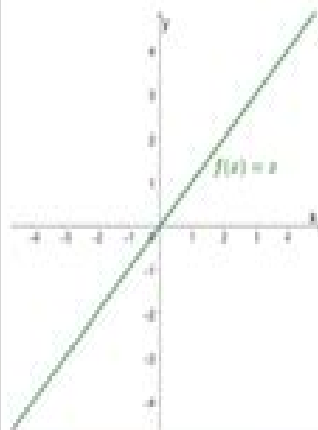
Linear Function
