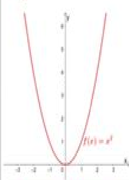
Quadratic Function
