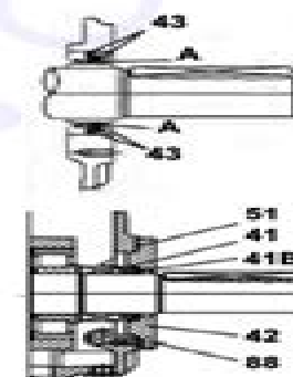
11.4 Sección RBS 135-225
