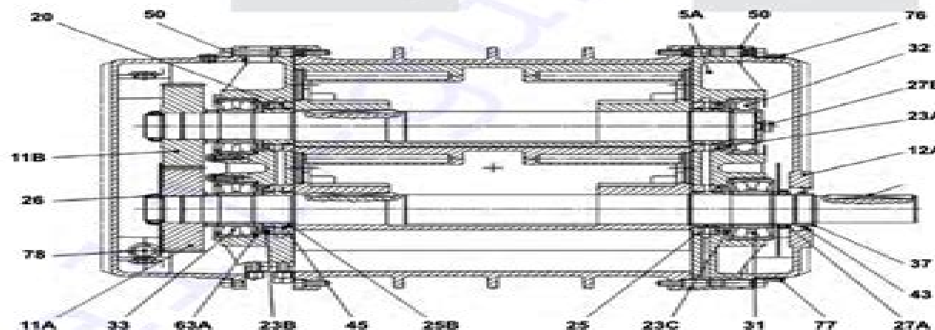
11.4 Sezione RBS 135-225
