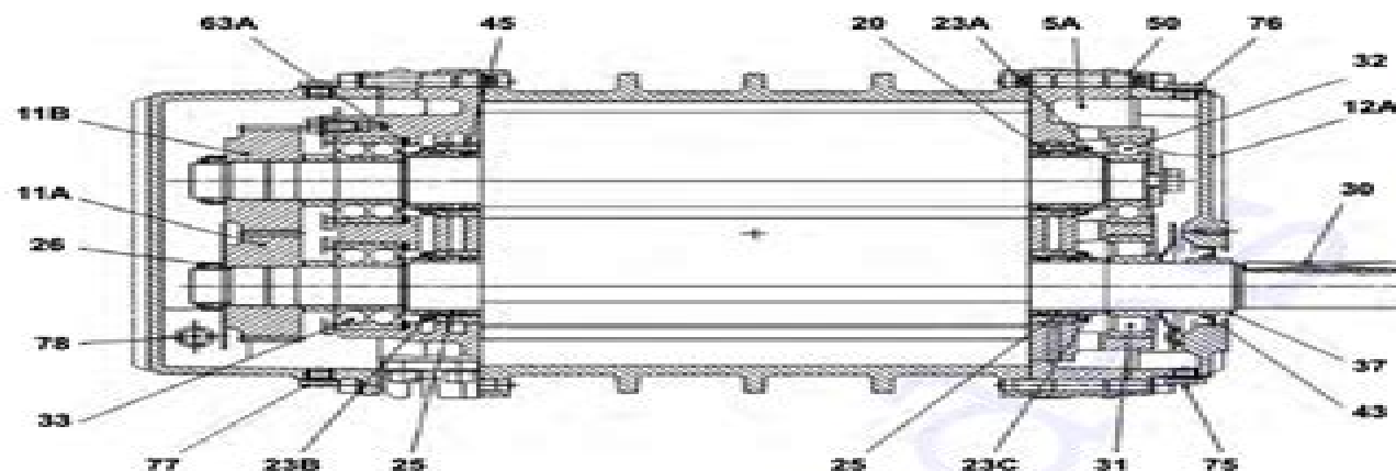
11.4 Sezione RBS 135-225
