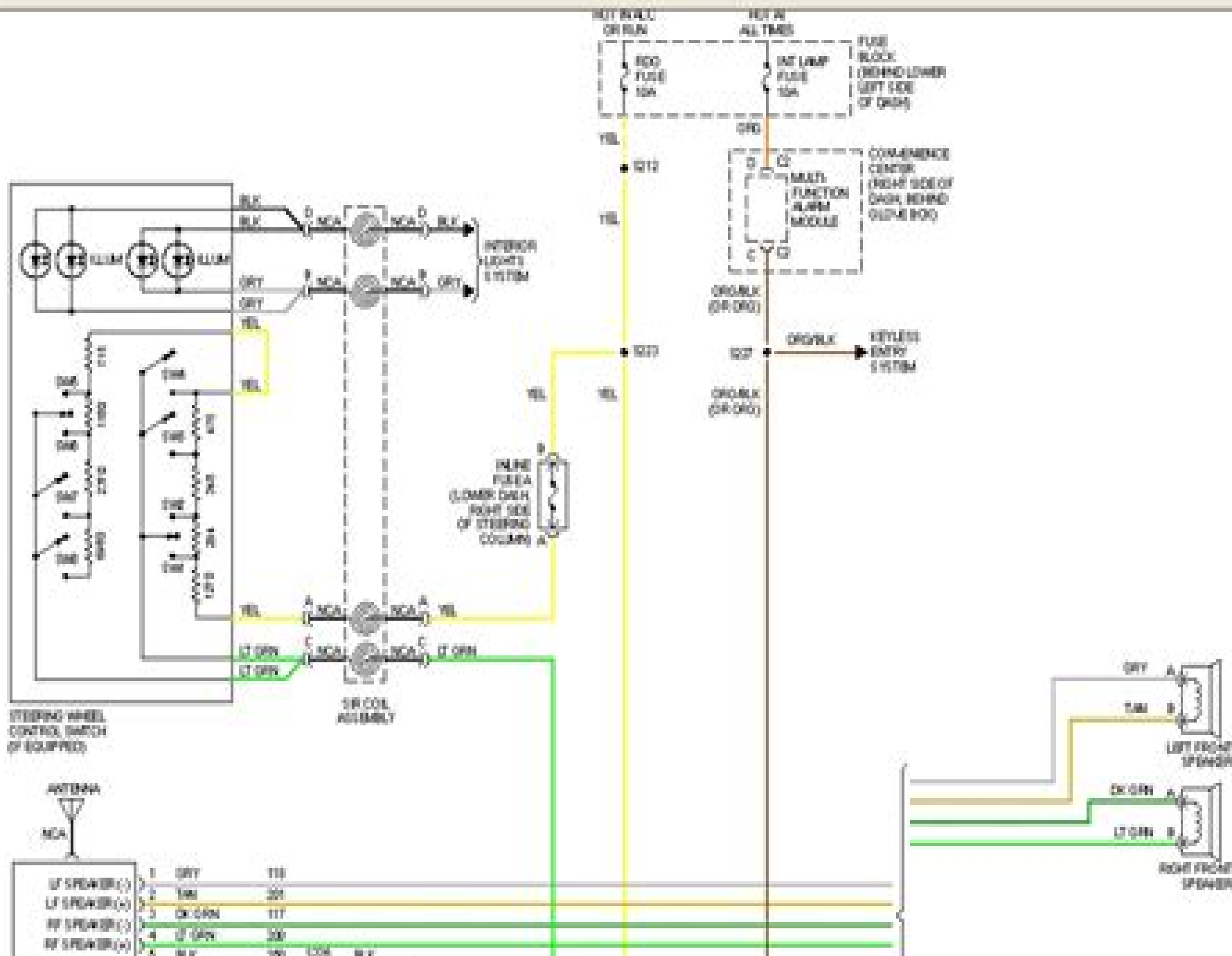
Fig. 34 Radio Circuits
