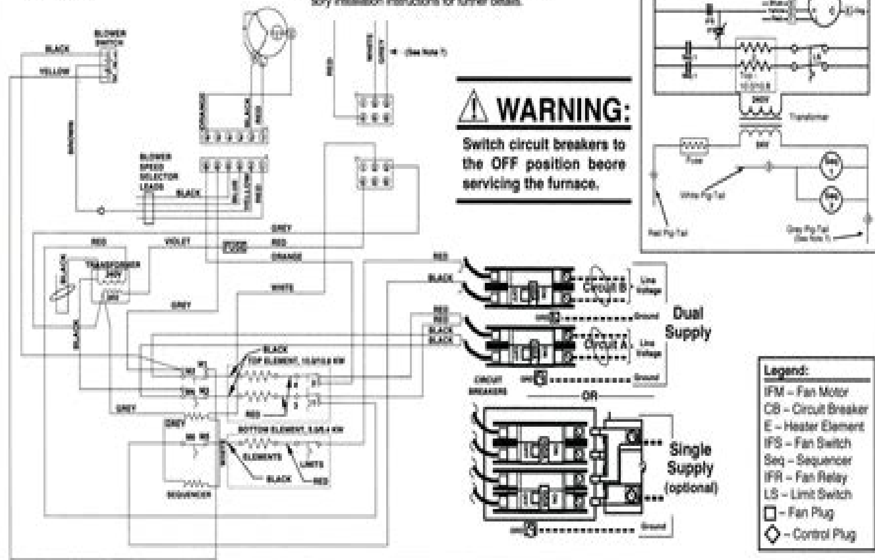
Figure 22. E2EH 015, 017 Wiring Diagrams
