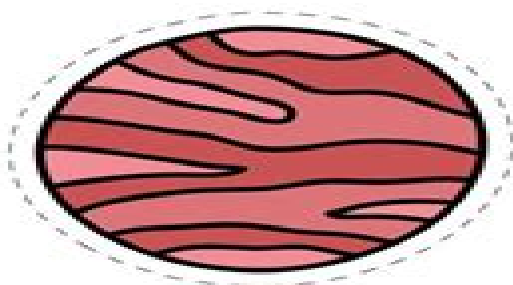
Venus
