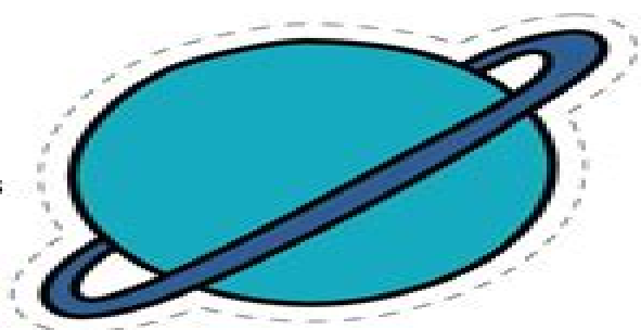
Uranus
