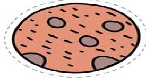
Mars
