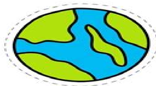
Earth
