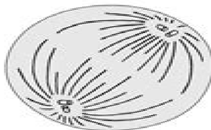
Metaphase I
