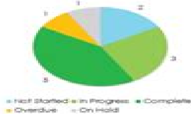
TASK STATUS %
