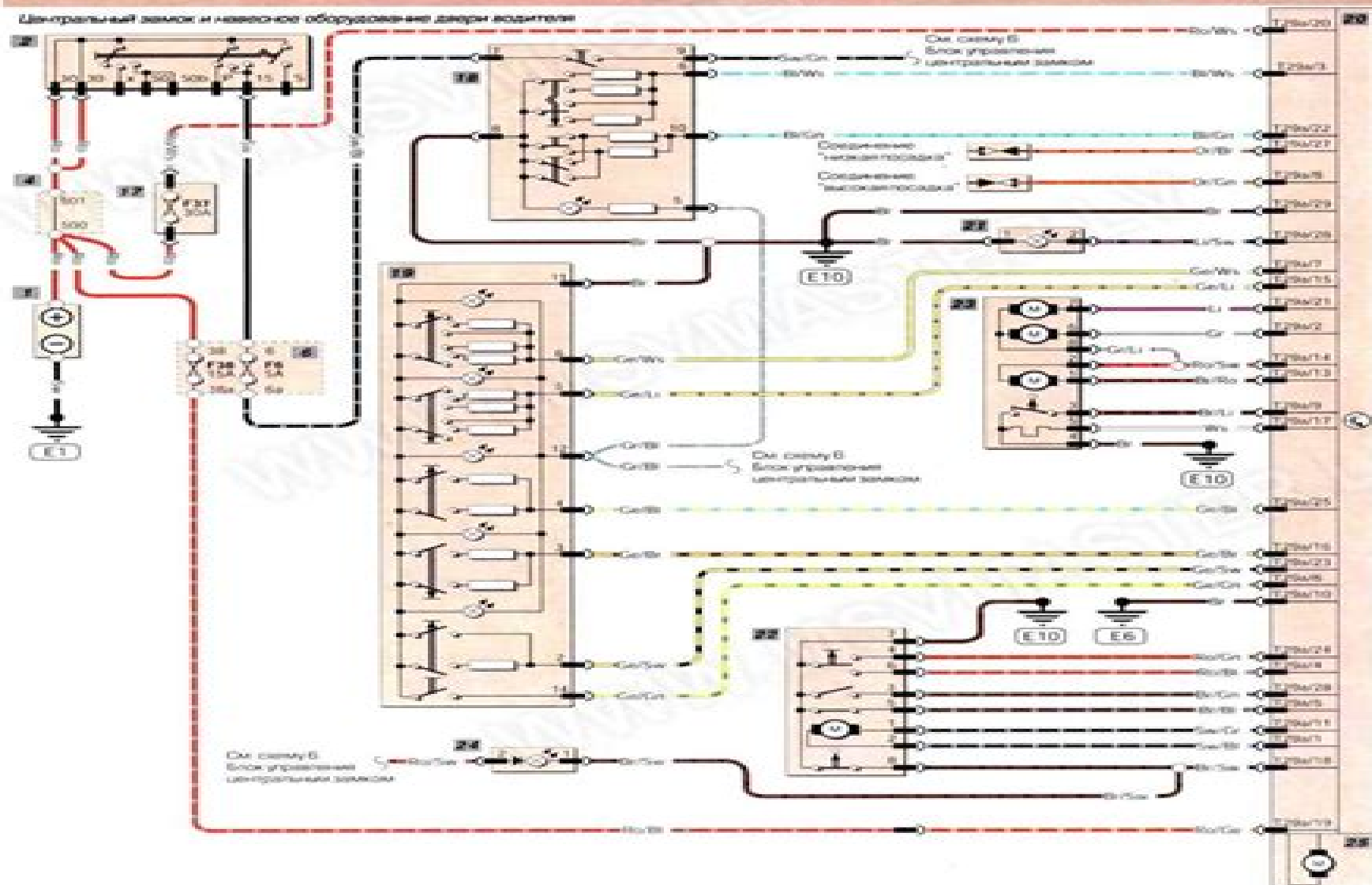
Центральный замок и навесное оборудование двери водителя
