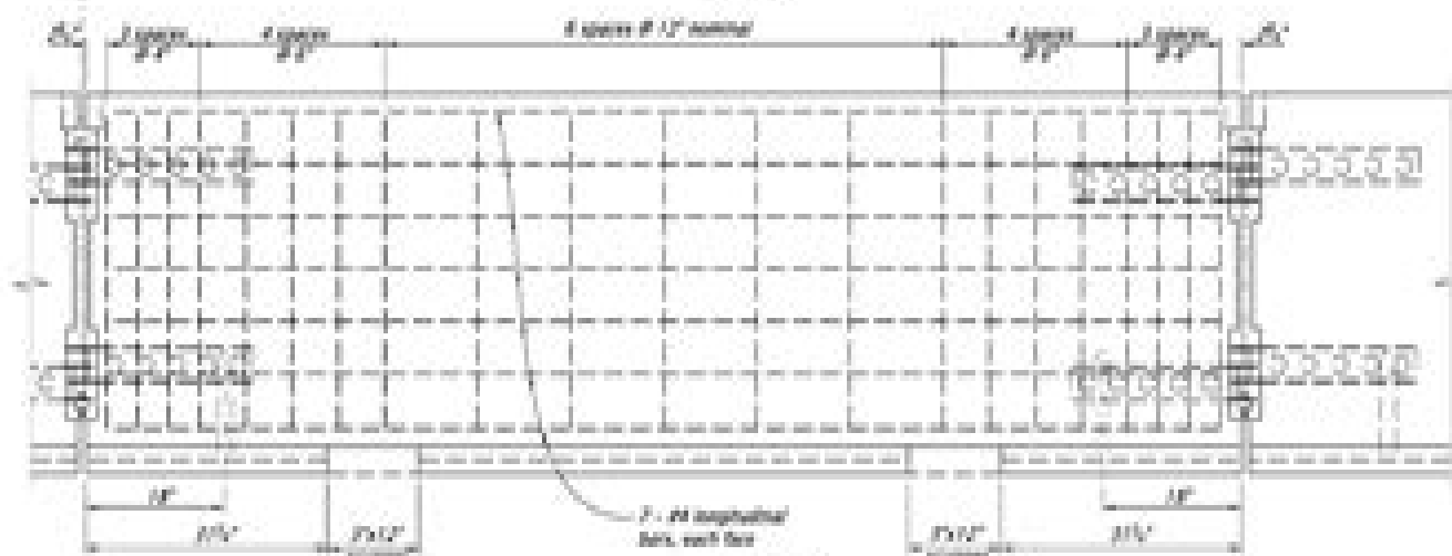
ELEVATION
