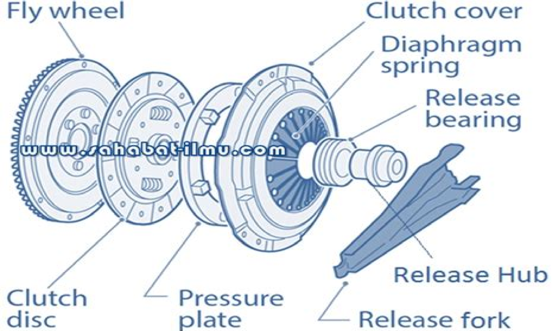
Bagian dari Kopling Gesek Plat Tunggal
