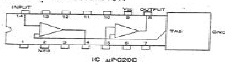
IC \mu PC20C
