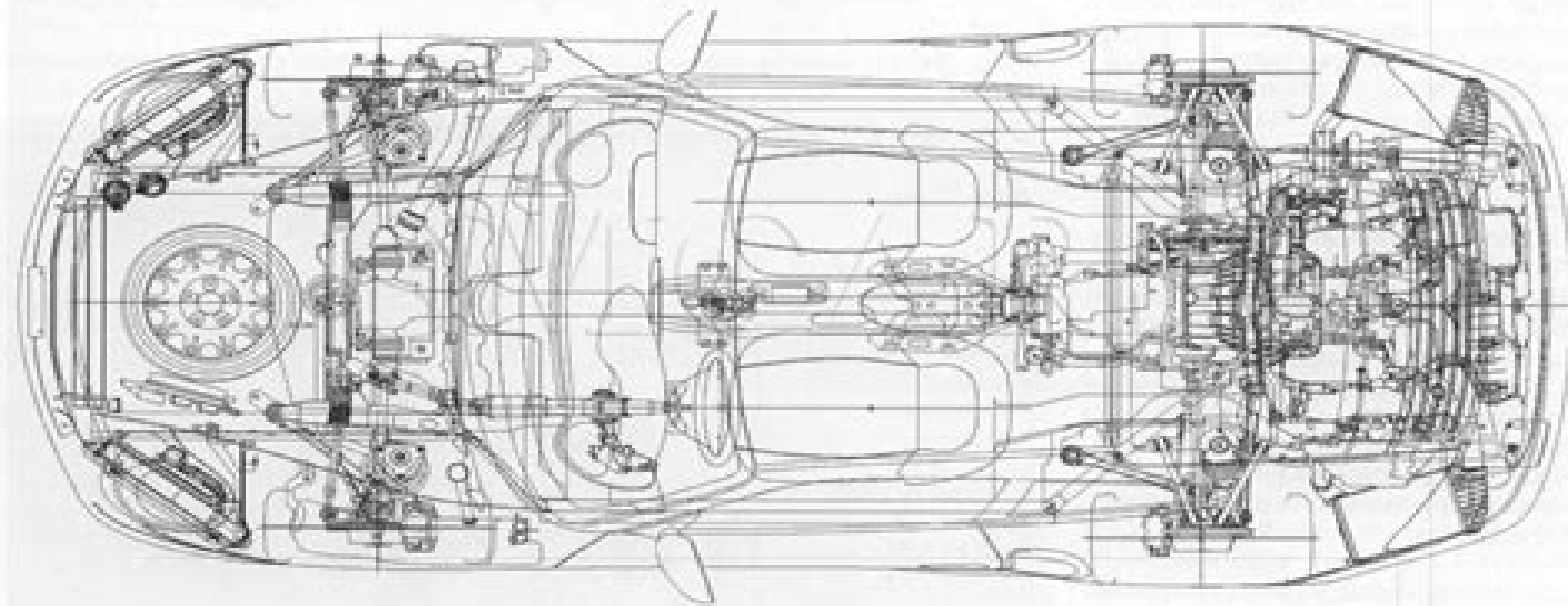
Bild 5: Package Draufsicht
