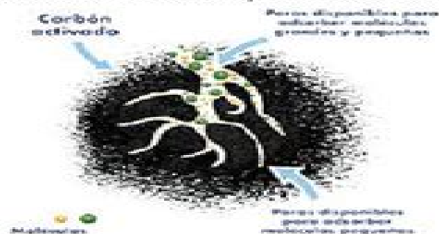
Figura 2. Adsorción de moléculas por carbón
