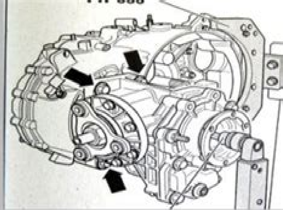
Abb. 5: Antriebswelle 5./6. bis Auslassventil einbauen
