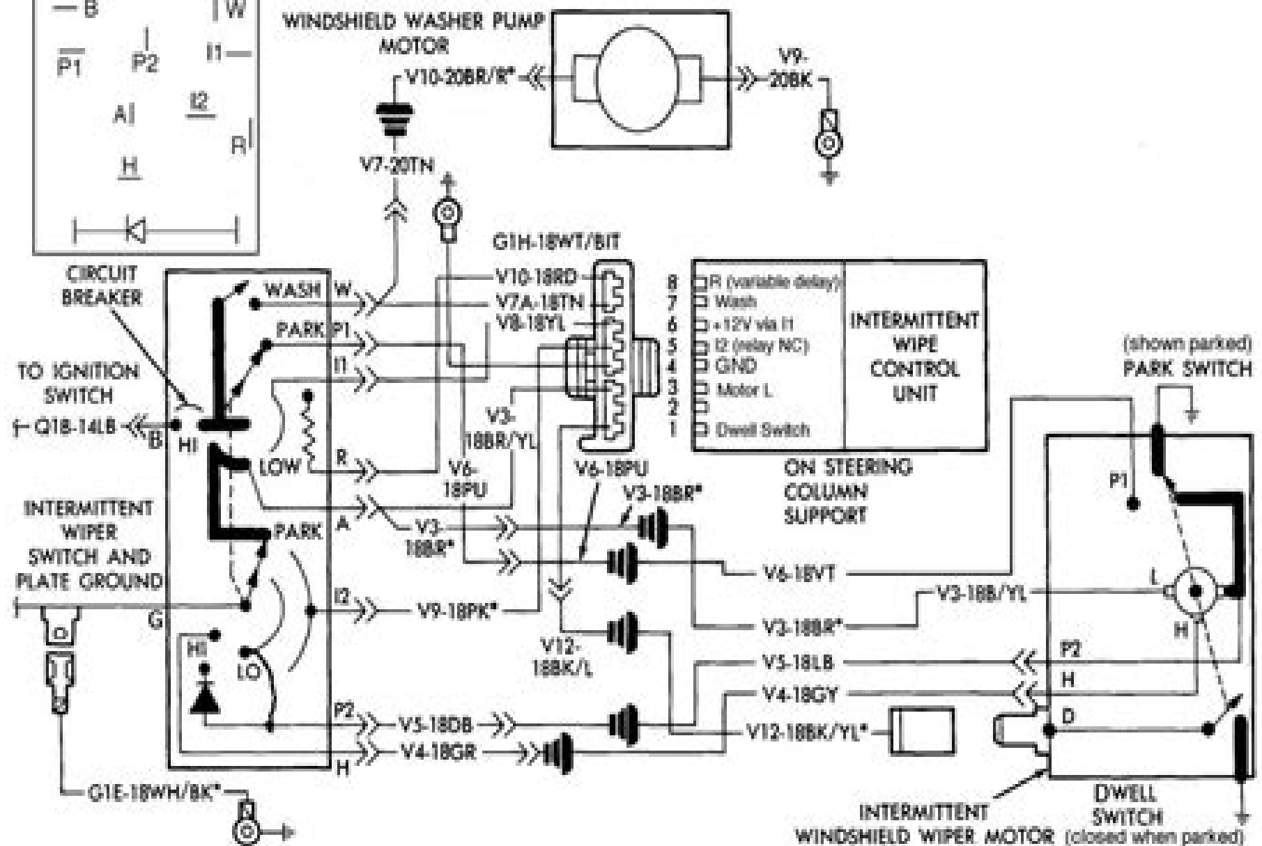
Fig. 25—Intermittent Wipe Wiring Schematic
