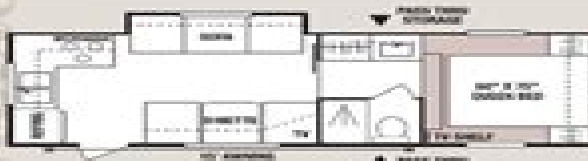
2352P-F - UVW 5530 - Dry Hsch Wt. 900 - NOC 1470 - Length 24'9"
