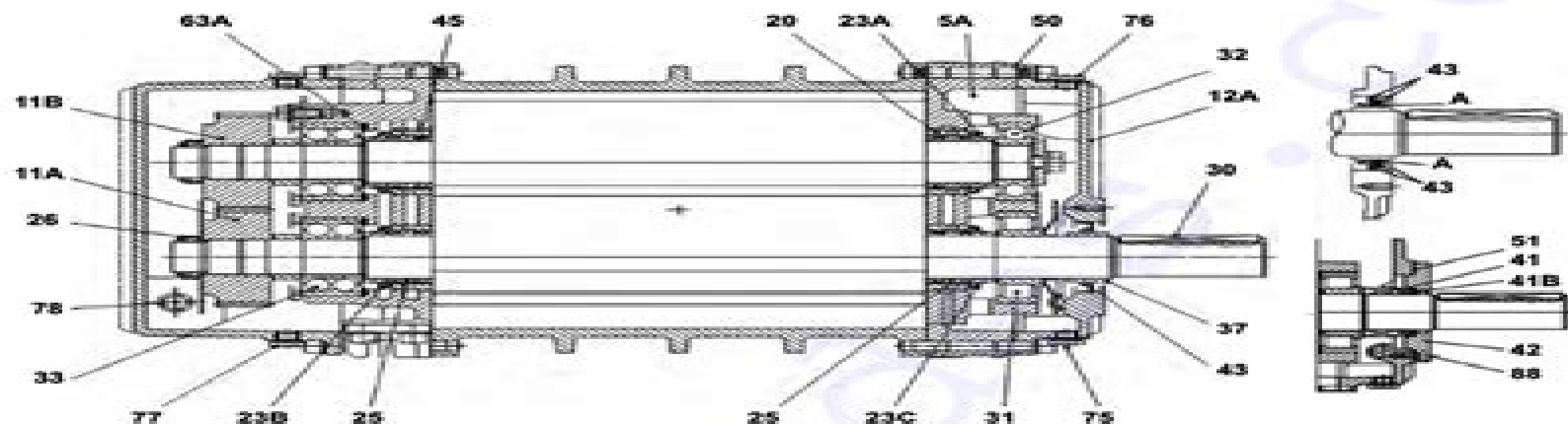
11.4 Sezione RBS 135-225
