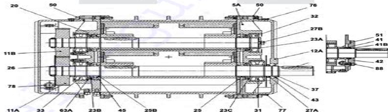
11.4 Sezione RBS 135-225
