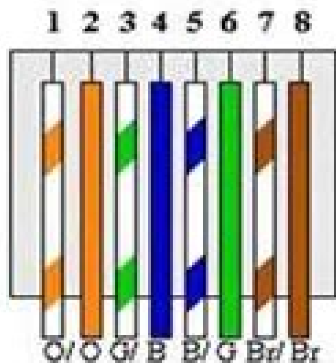
T-568B
