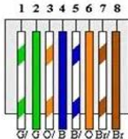
T-568A
