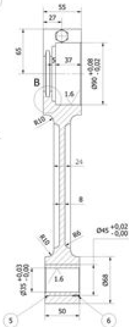
A-A (1 : 2)
