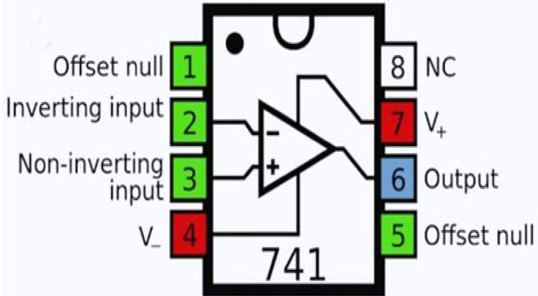
741 IC Pinout
