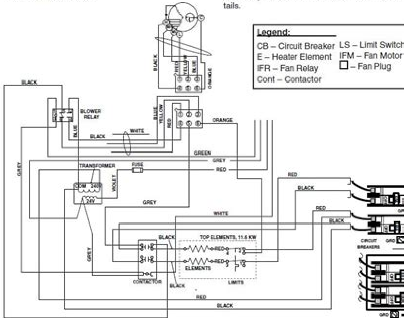
Figure 27. E3EB 012H Wiring Diagrams
