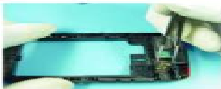
27. Remove the CONN ANT.
