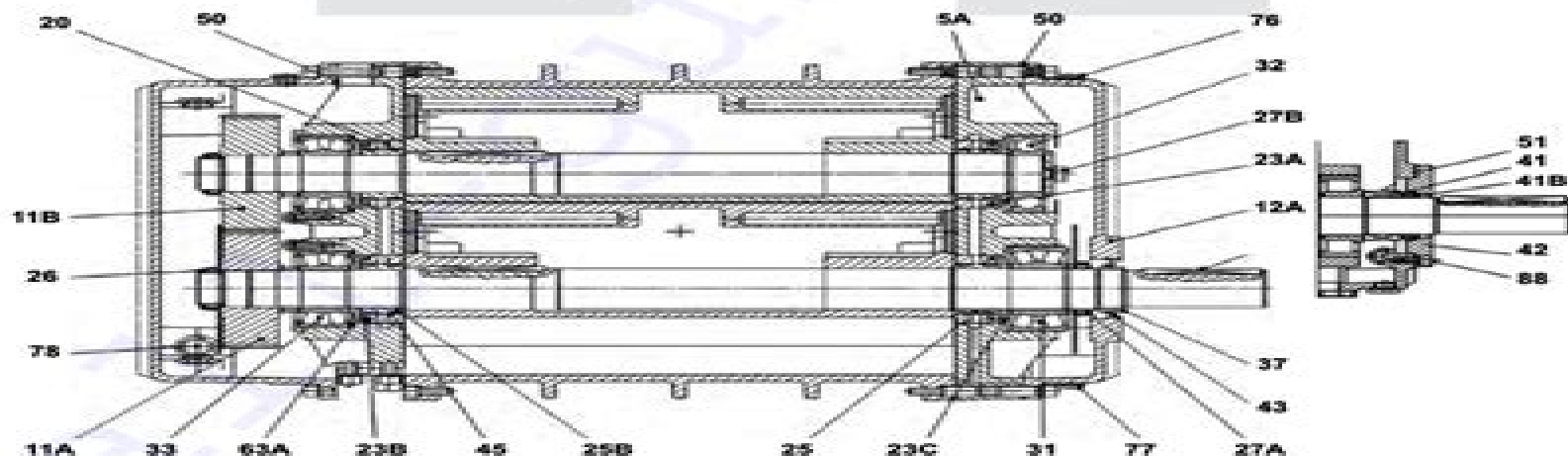
11.4 Sezione RBS 135-225
