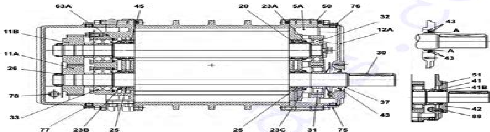
11.4 Sezione RBS 135-225
