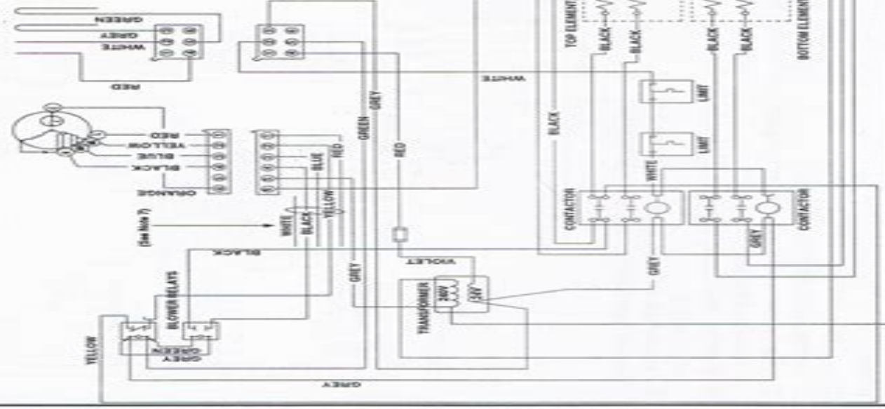
Figure 30. E2EB 020, 023, and 023 - 5 Ton Wiring Diagrams
