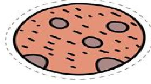
Mars
