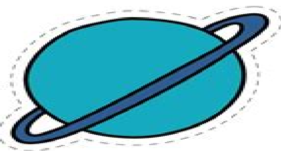
Uranus
