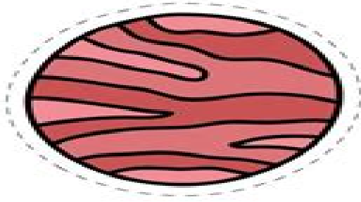
Venus
