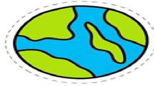
Earth
