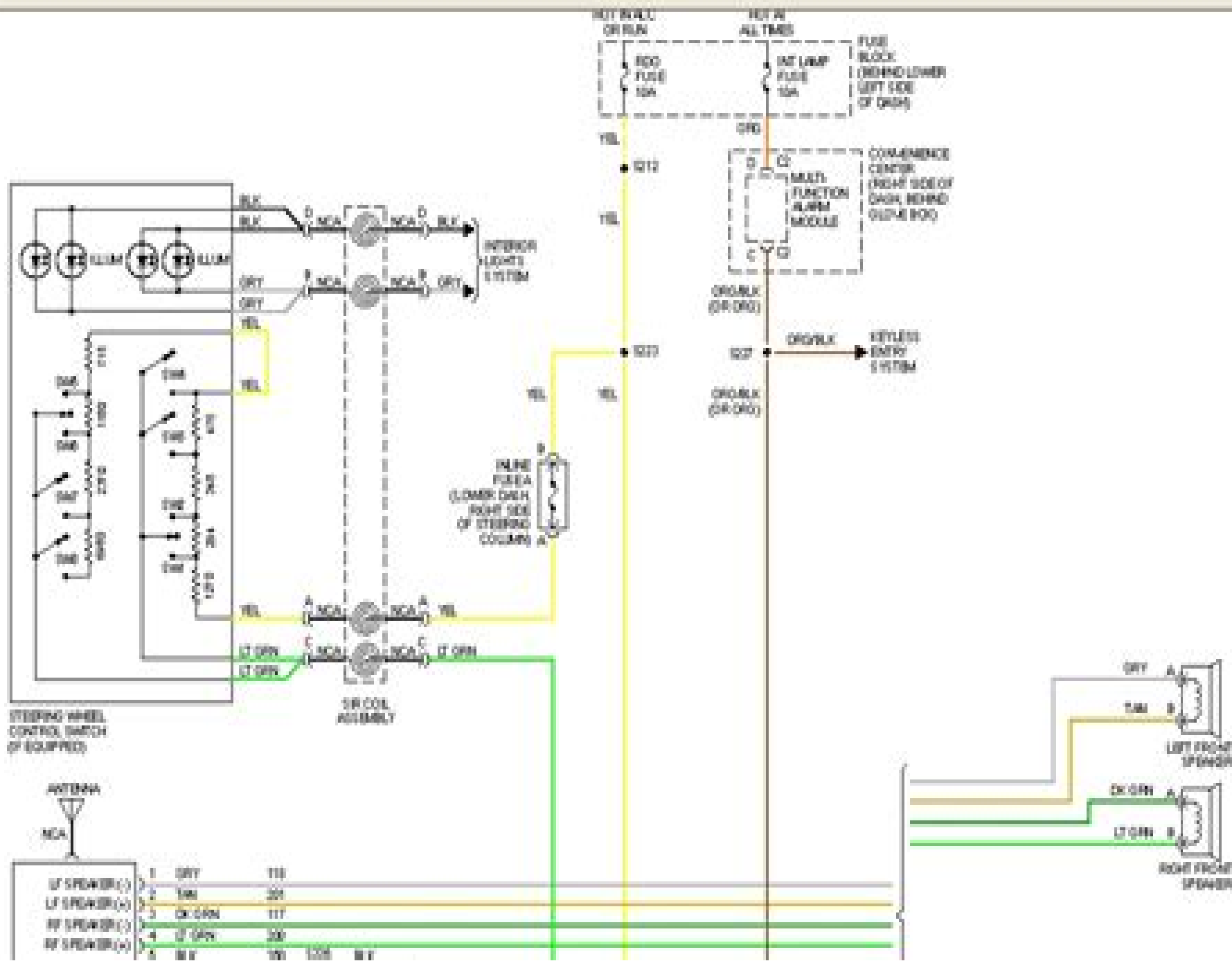
Fig. 34 Radio Circuits
