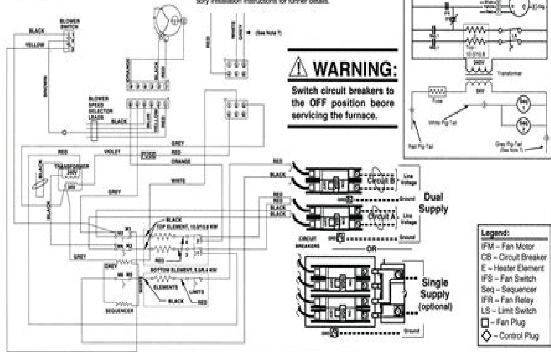
Figure 22. E2EH 015, 017 Wiring Diagrams
