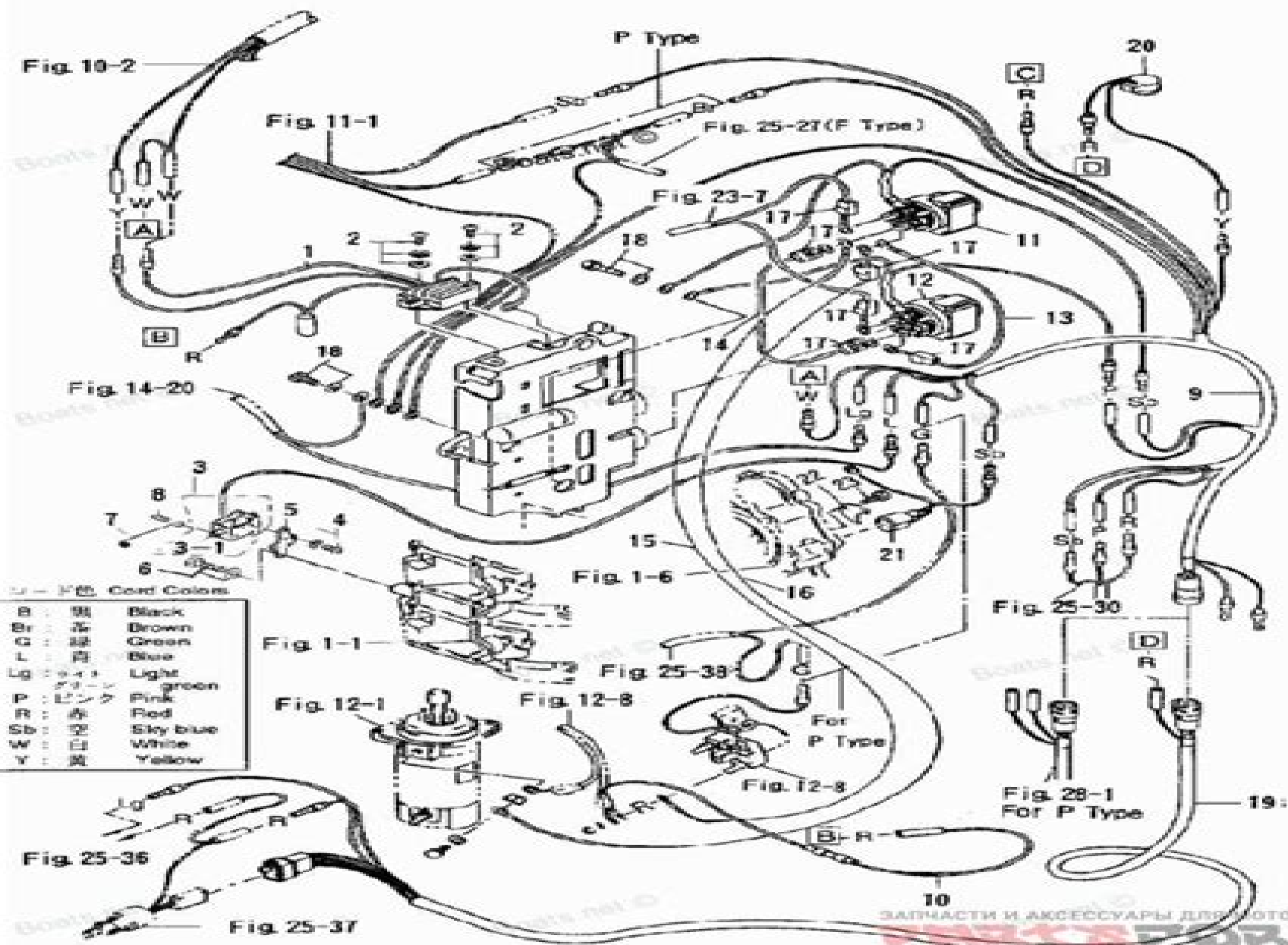
Fig. 13 エレクトリックパーツ (ダイアグラム : E タイプ) ELECTRIC PARTS (DIAGRAM : E Type)
