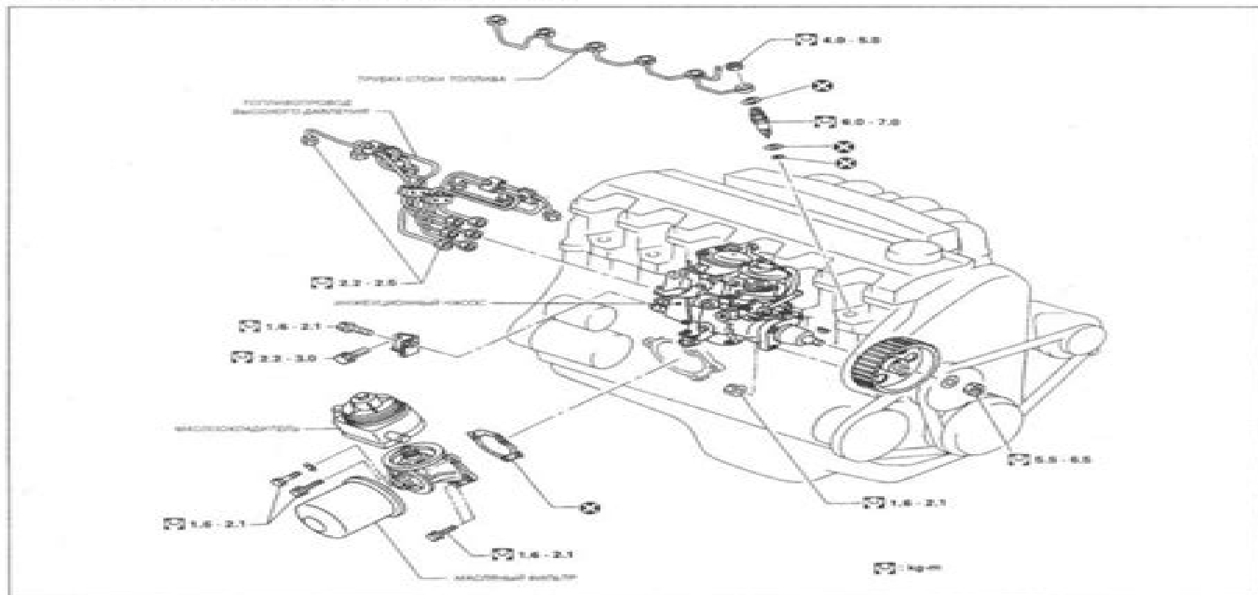
Рис. 3-1. Внешние компоненты RD28T — правая сторона.
