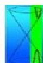
Hyperbola
