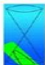
Parabola
