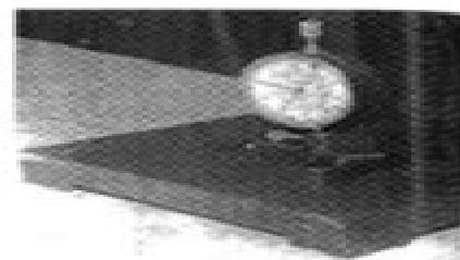
Montaje del comparador para medir la altura de las camisas.
