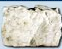
34. Gypsum
