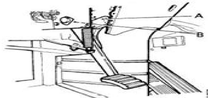
Interruptor del pedal del embrague
