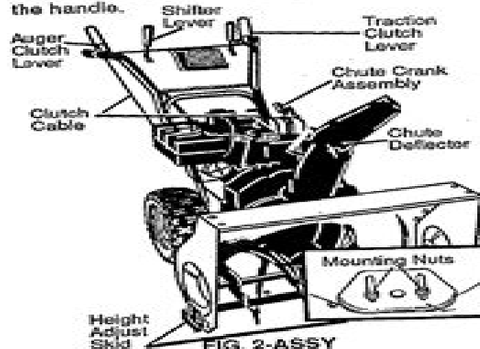
FIG. 2-ASSY
