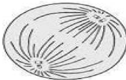
Metaphase I
