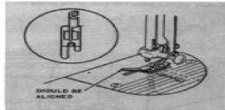
Fig. 9. Aligning Presser Foot
