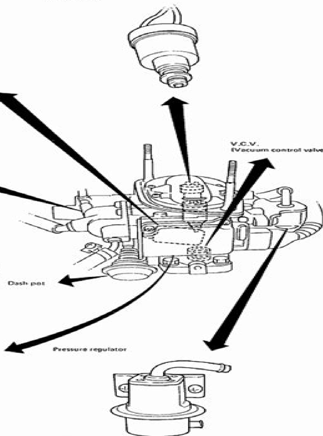
Injector (X2)
