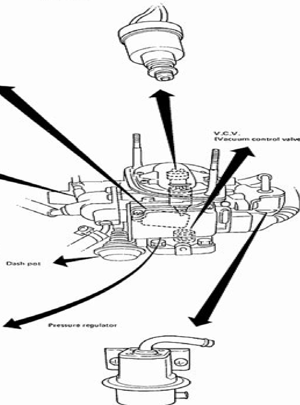
Injector (X2)
