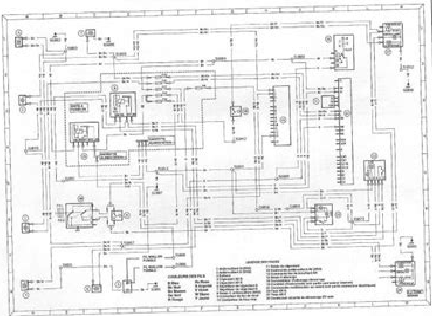
Schéma 26 / Schéma électrique - four stop, de nuit, de freinage et direction
