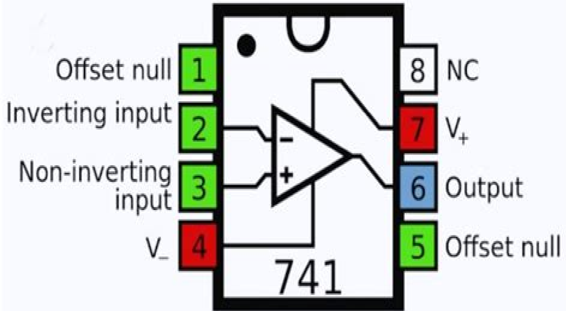
741 IC Pinout
