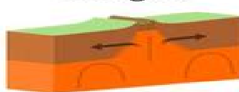
Divergent
