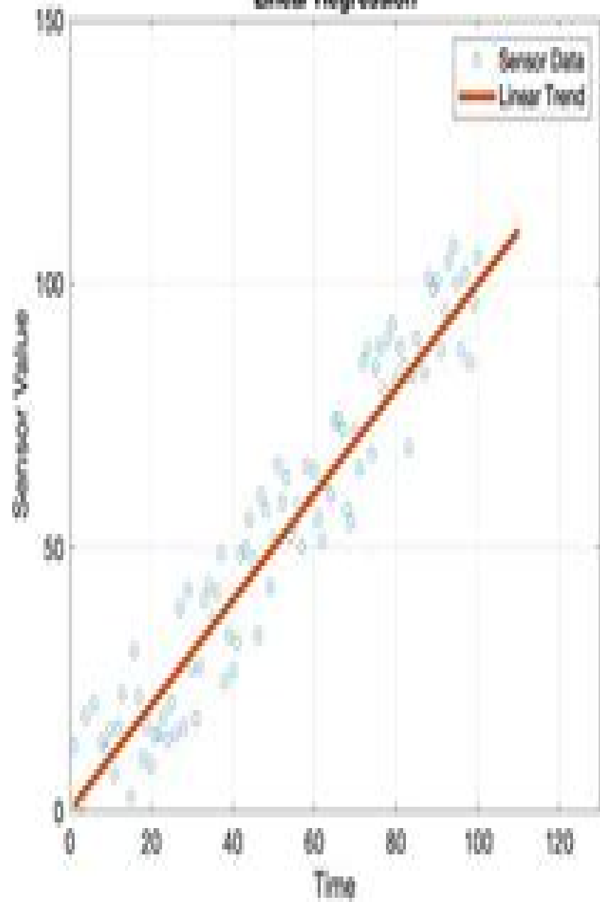
Linear Regression
