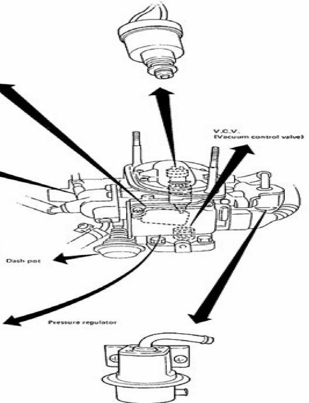
Injector (X2)
