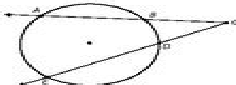
Secant-secant
