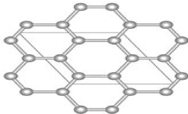
Anti-KekuléGr
