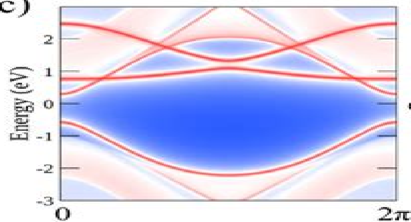
Anti-KekuléGr
